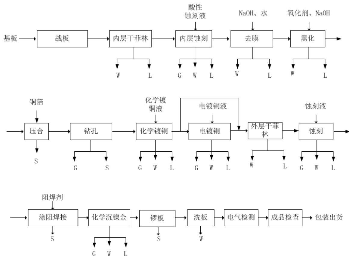
图 2.2-1 生产工艺流程图
