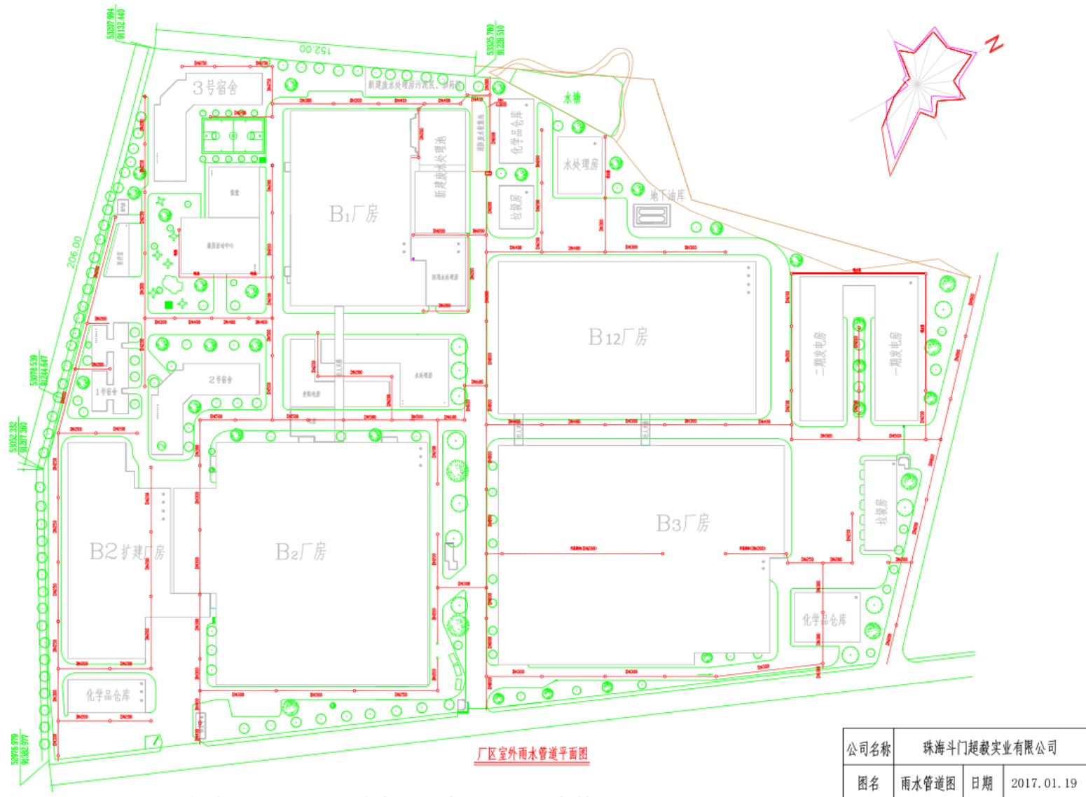
附图 5 室外雨水管网图
