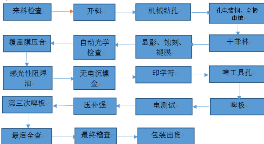
三、软硬结合板工艺流程图：
